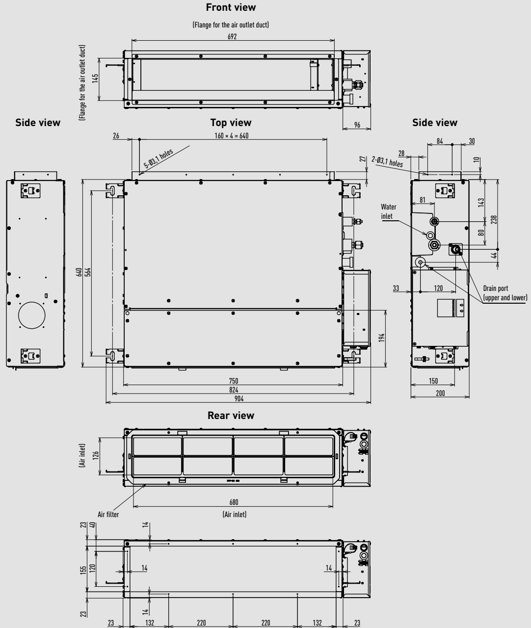
CU-Z25UBEA
